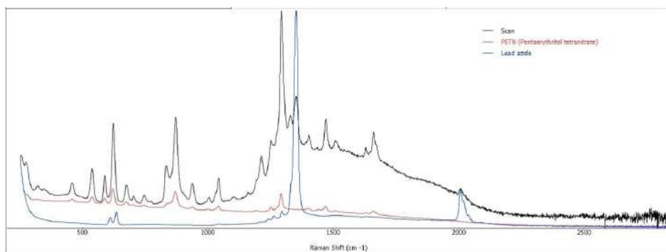
Figure 5: Spectre d'un mélange de PETN 82% et azoture de plomb 3%
