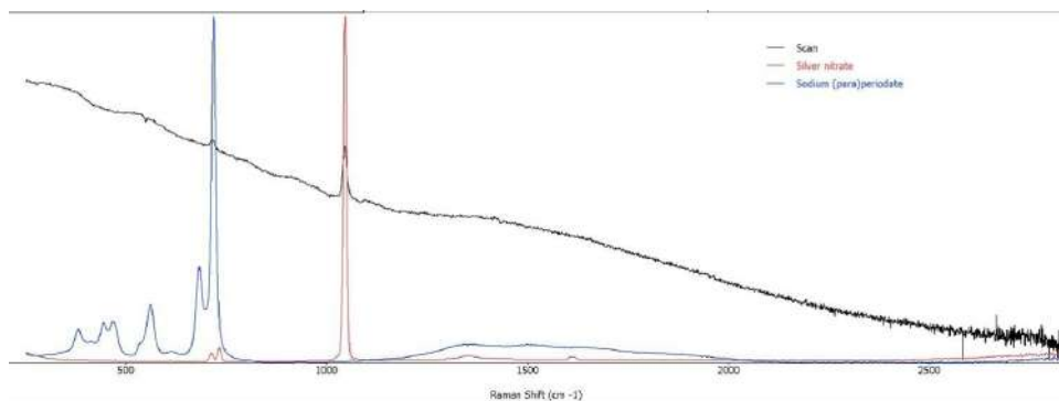
Figure 6: Spectre d'un mélange de Nitre d'argent 86% et (para) périodate de sodium 3%)
